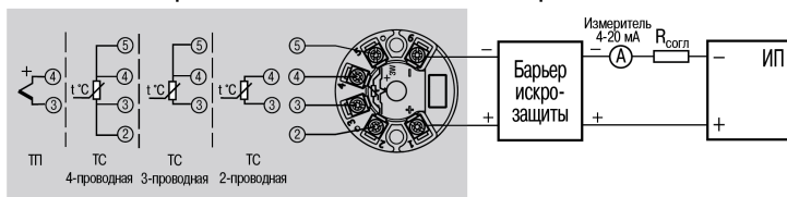
Рисунок 6.3 – Подключение прибора
