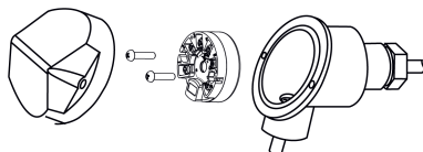
Рисунок 6.2 – Монтаж прибора
